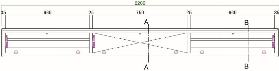
【 220AVボード正面/内部図】
