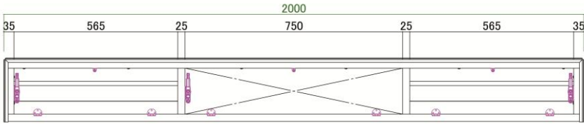
【 200AVボード正面/内部図】
