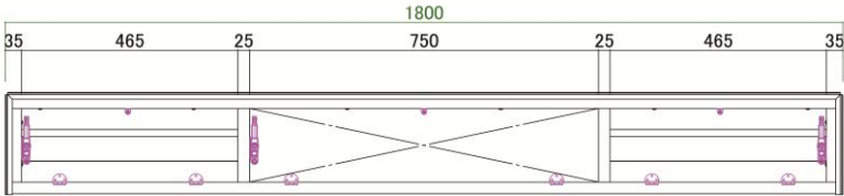
【 180AVボード 正面/内部図】
