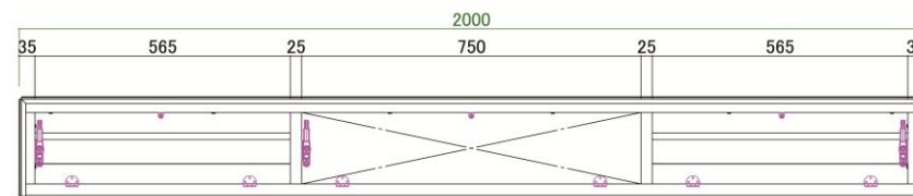
【200AVボード 正面/内部図】
