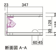
断面図 A-A
