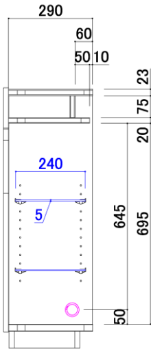
断面図 A-A
