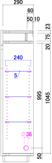
断面図 B-B
