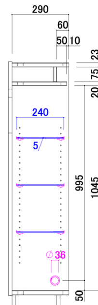
断面図 A-A
