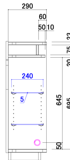
断面図 A-A
