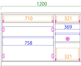
●120サイドボード正面図
