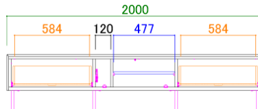
●200AVローボード正面図
