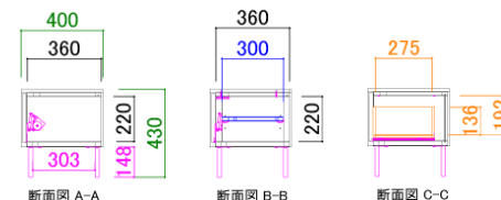
●AVローボード共通断面図
