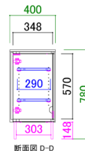
●サイドボード共通断面図
