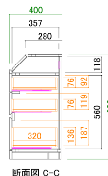
40 chests 断面図
