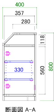
80サイドボード 断面図
