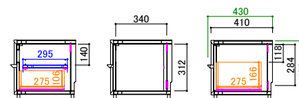
AV ローボード 断面図
