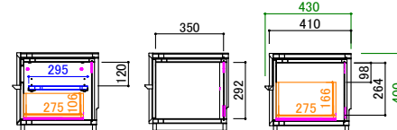
240 AV ローボード 断面図
