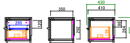
240 AVローボード 断面図
