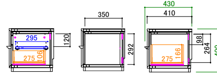
240 AV ローボード断面図
