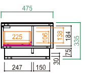
断面図 F-F
