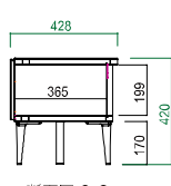
断面図 C-C
