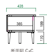
断面図 C-C
