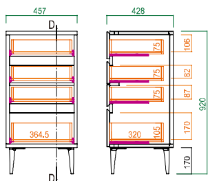
断面図 D-D
