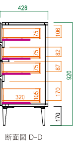
断面図 D-D
