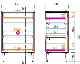
断面図 E-E
