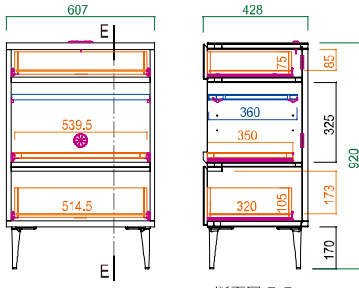
断面図 E-E
