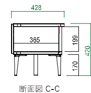
断面図 C-C
