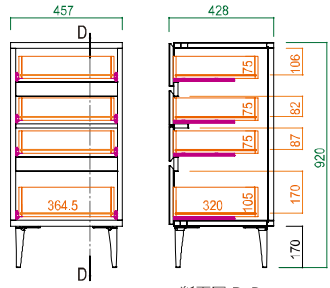
断面図 D-D
