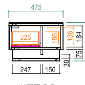
断面図 F-F
