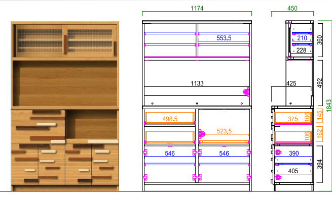
120キッチンボード サイズ: W1174 D450 H1843 定 価: ¥182,300 (税別)
