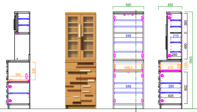
60ダイニングボード サイズ: W590 D450 H1843 定 価: ¥116,200 (税別)
