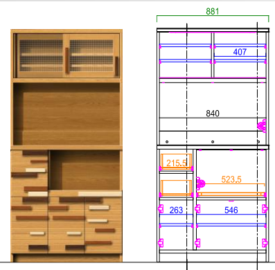
90キッチンボード サイズ: W881 D450 H1843 定 価: ¥151,900 (税別)
